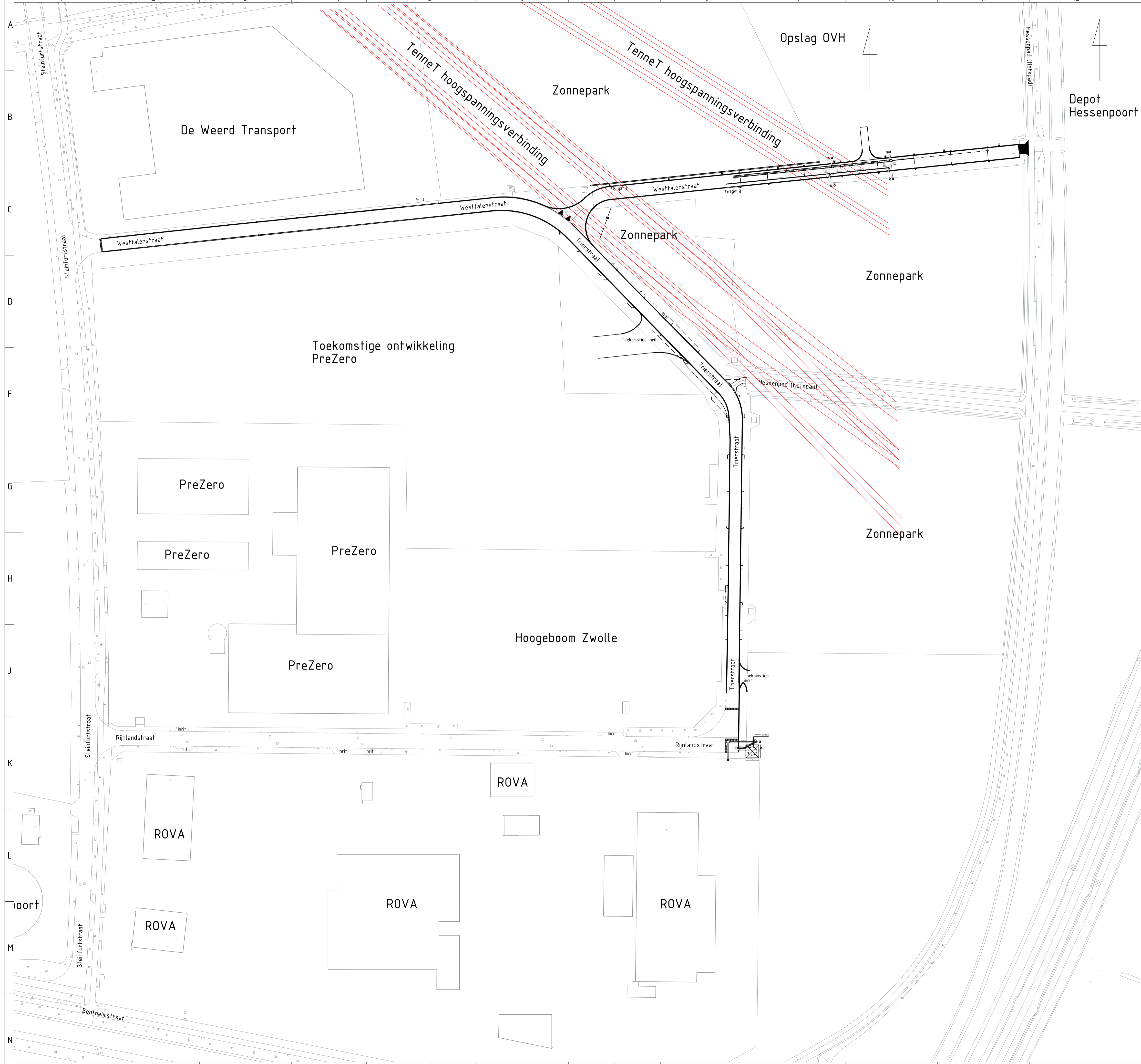
OVERZICHT HESSENPOORT Schaal 1:10000
