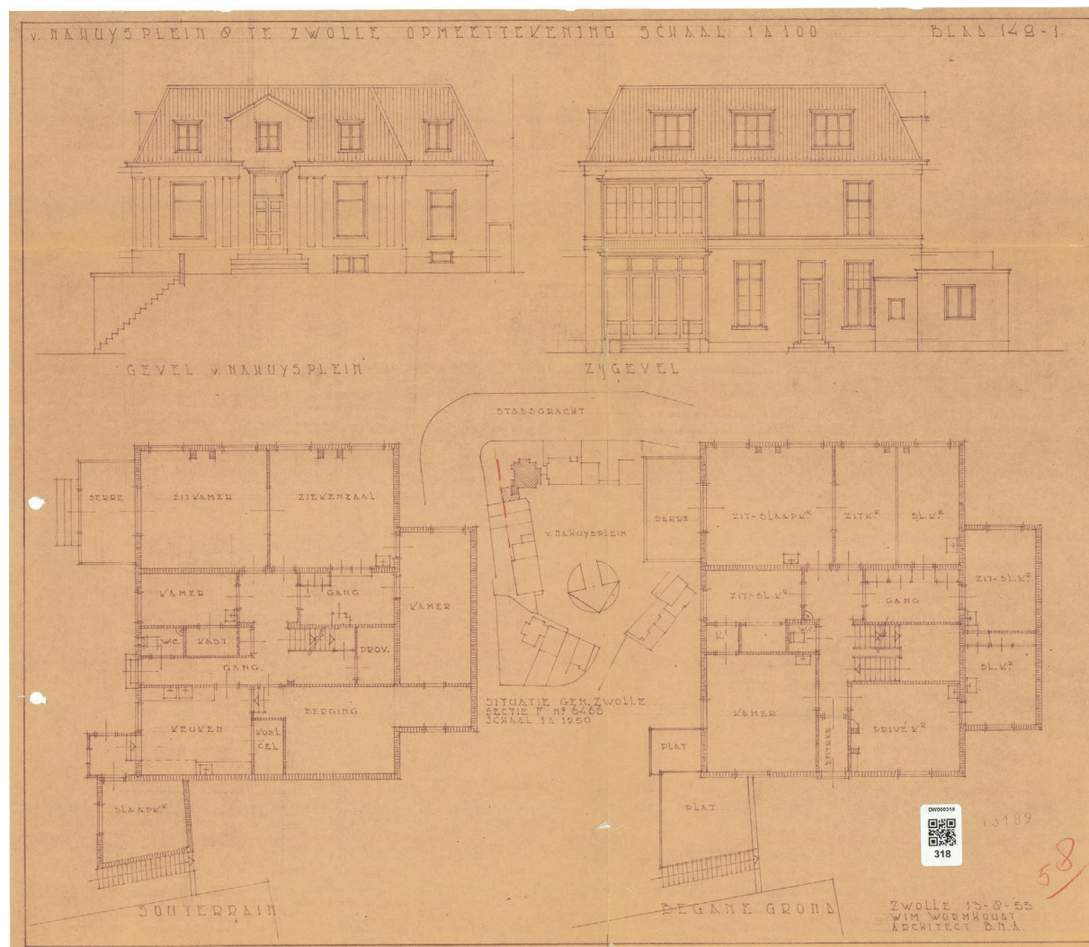
Plattegronden en gevelaanzichten en situatie, bestaand, 1955-56
