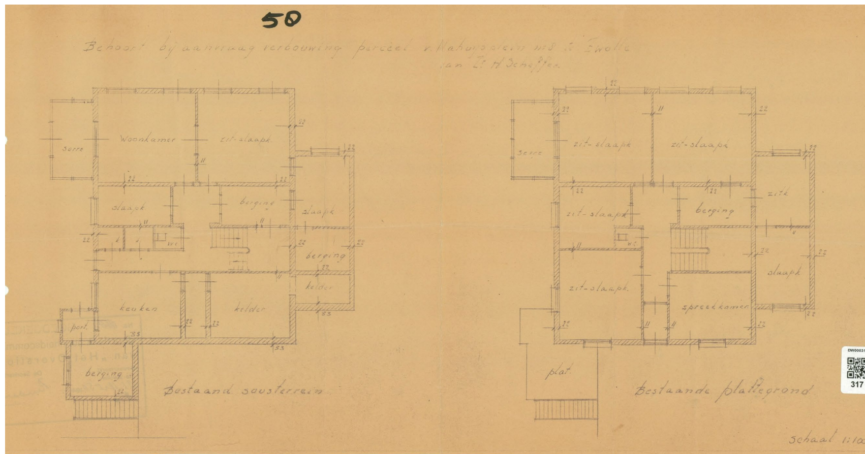
Plattegronden bestaande situatie, 1950
