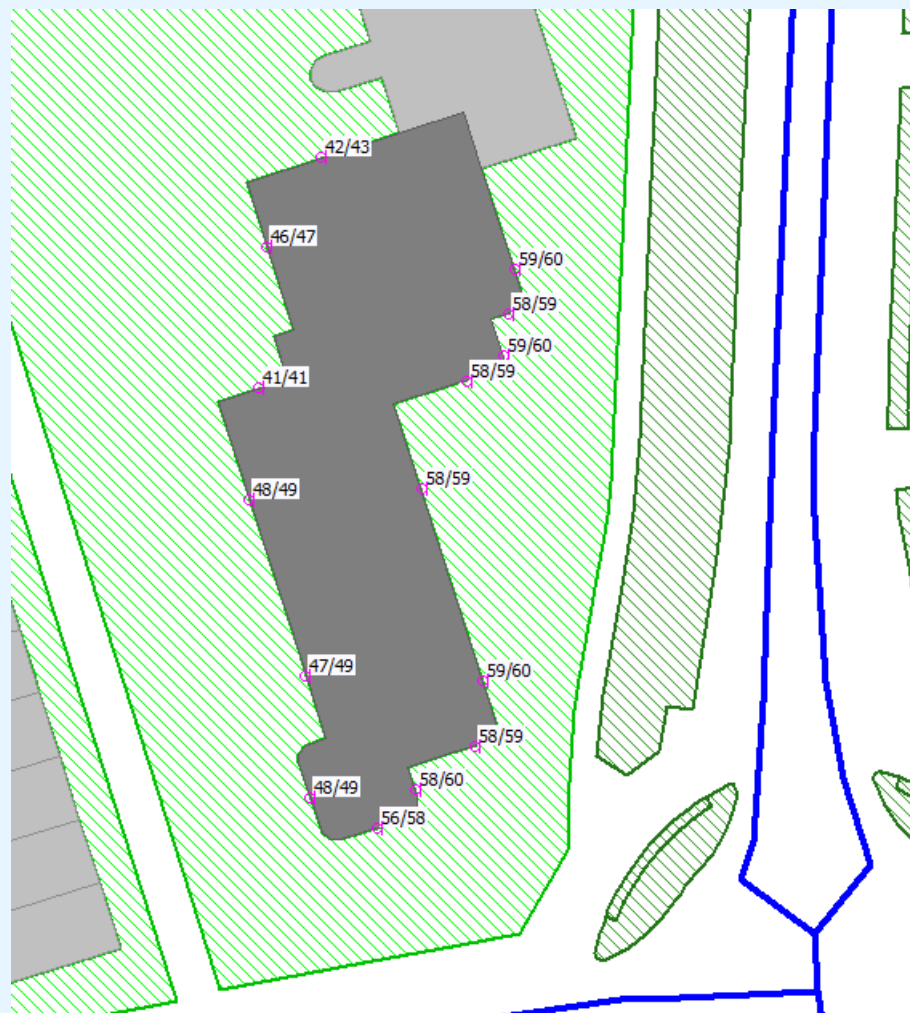
figuur 8: gezamenlijk geluid Lden van alle wegen Omgevingswet
