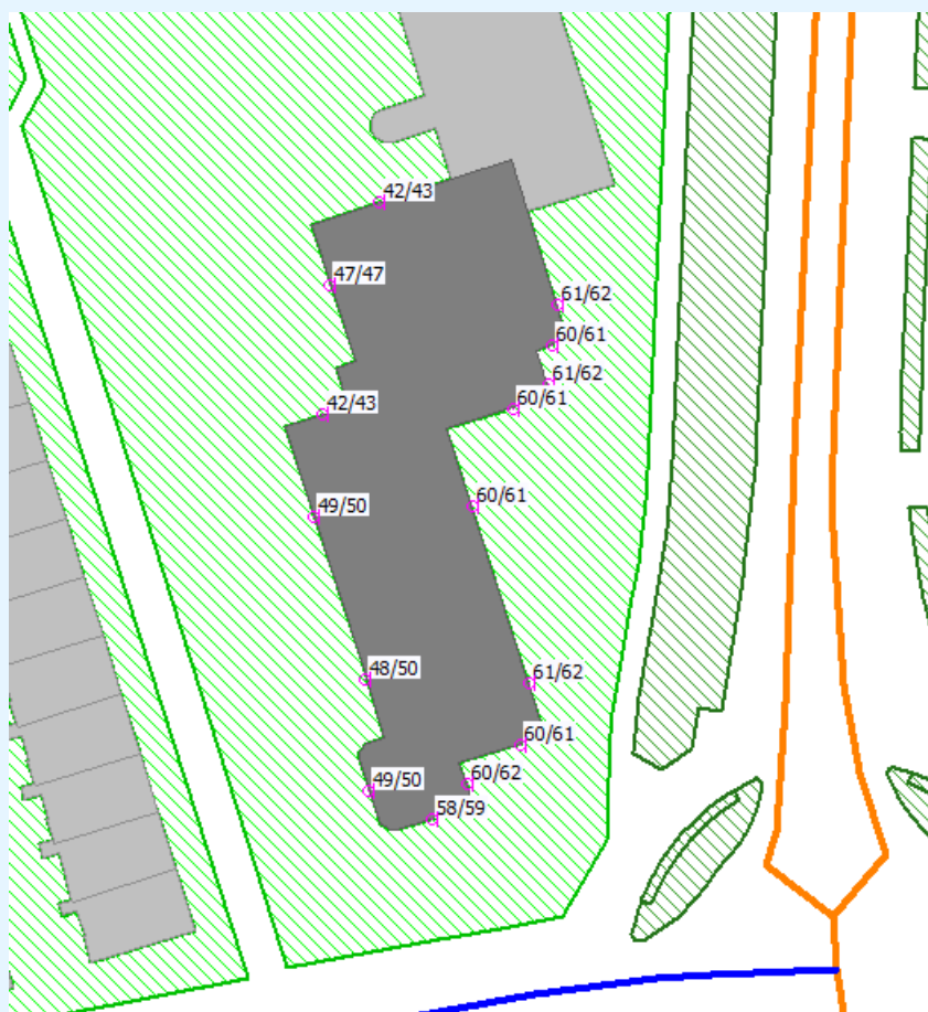
figuur 7: geluidsbelasting per bouwlaag vanwege alle wegen samen (excl. aftrek artikel 110 Wgh)
