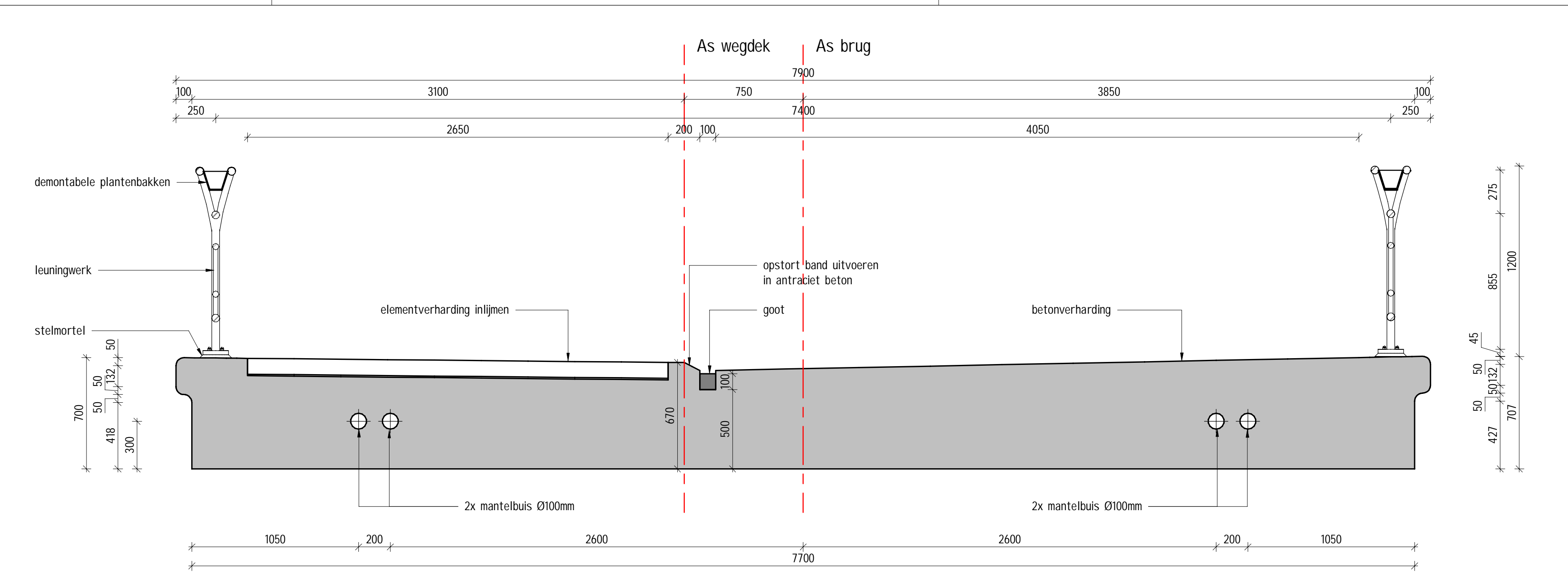
Dwarsdoorsnede D-D schaal 1 : 20
