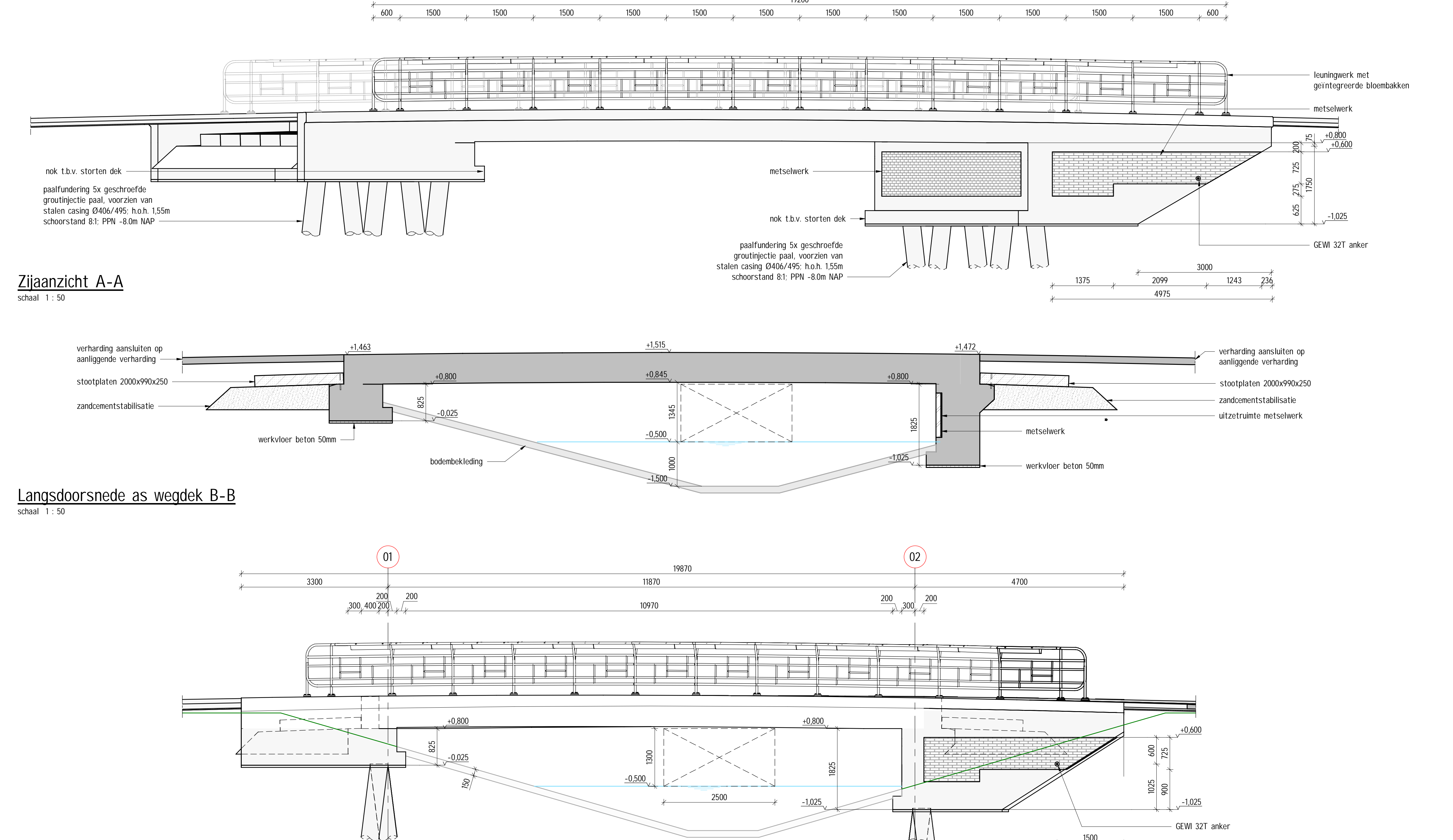
Zijaanzicht as watergang C-C schaal 1 : 50
