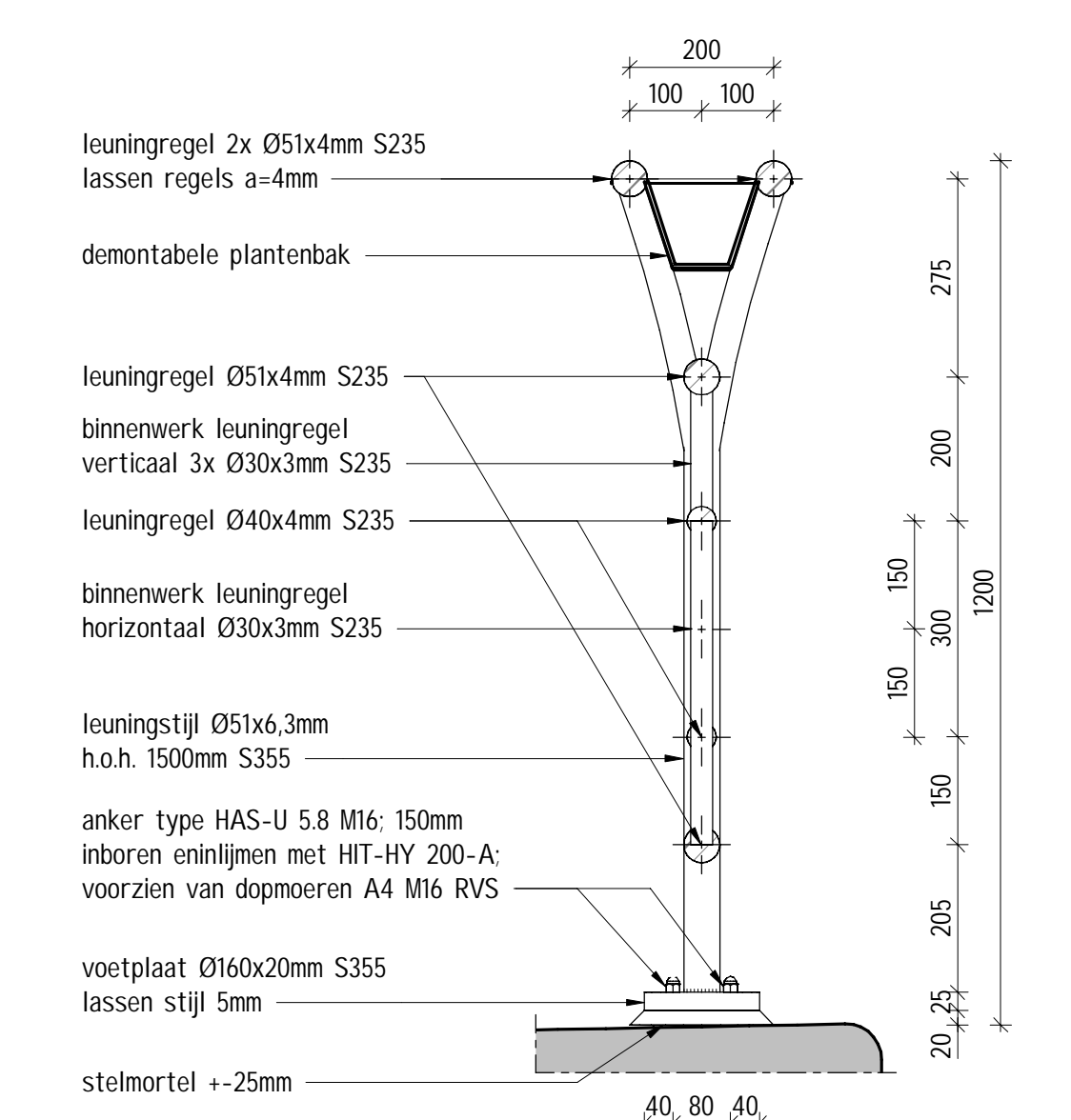
Detail 01 - Leuningwerk schaal 1 : 10
