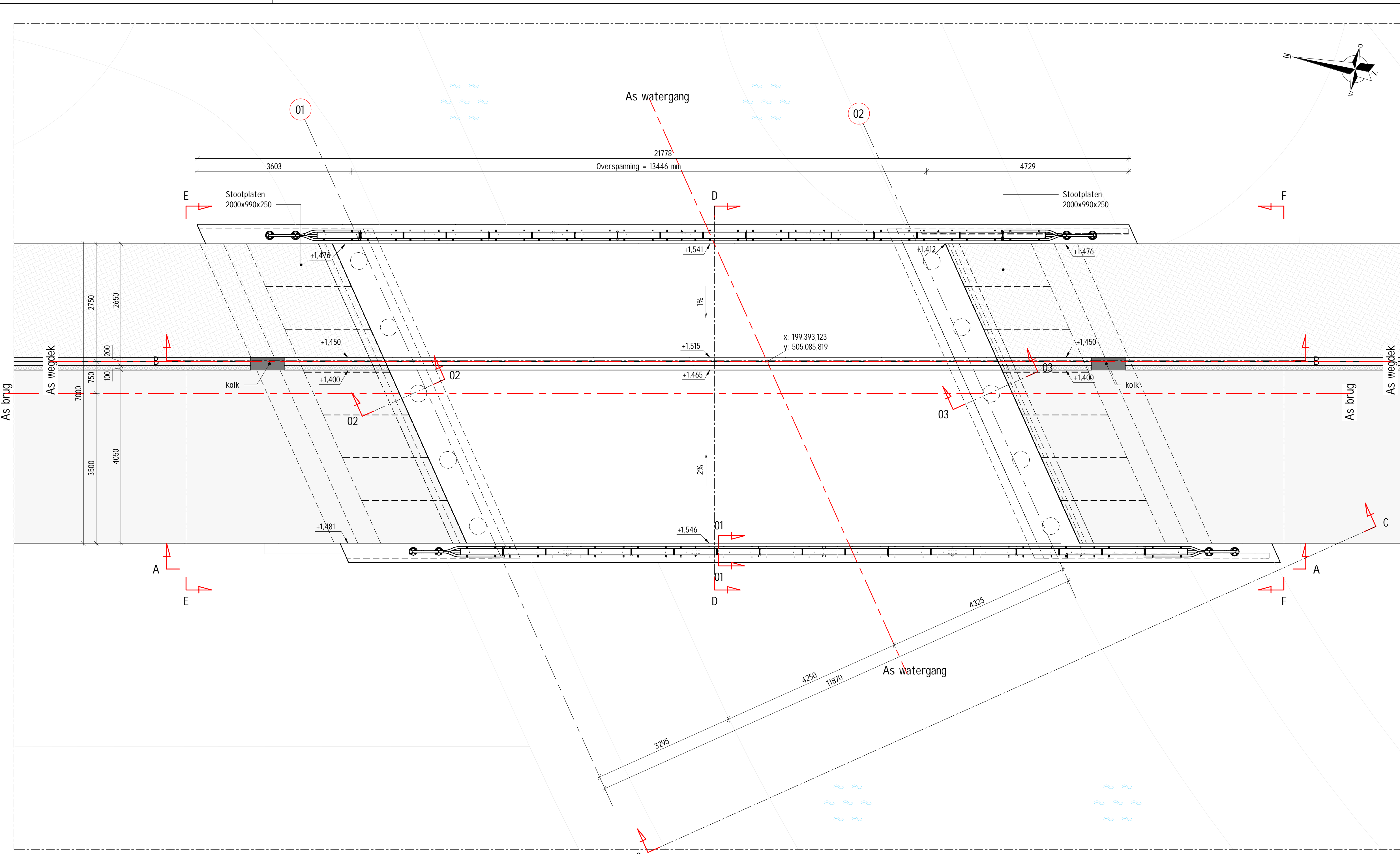
Bovenaanzicht schaal 1 : 50
