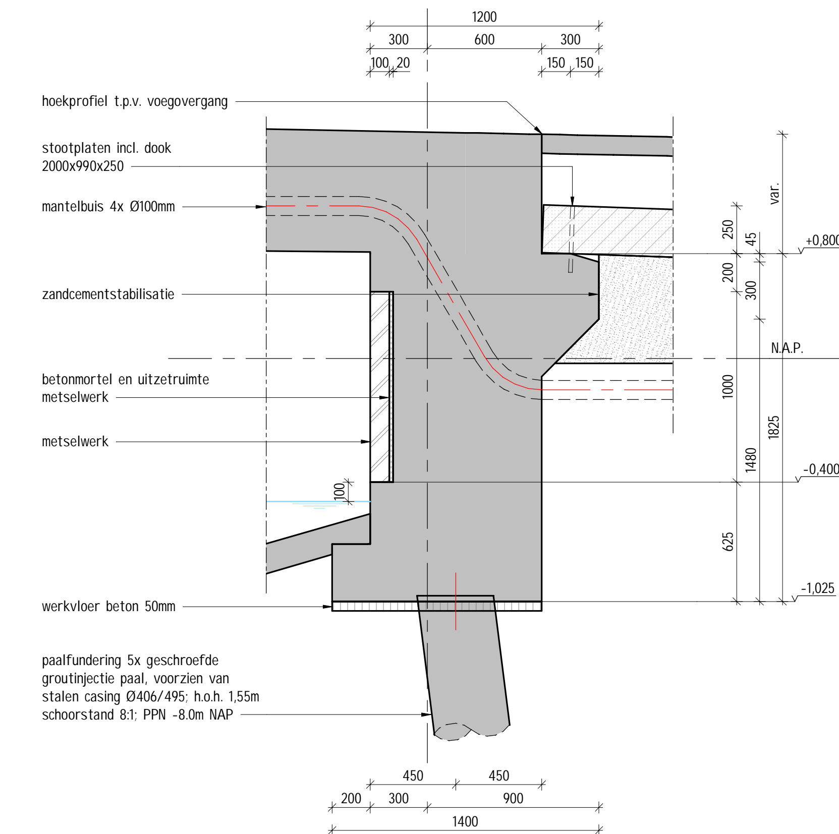
Detail 03 - landhoofd zuid schaal 1 : 20
