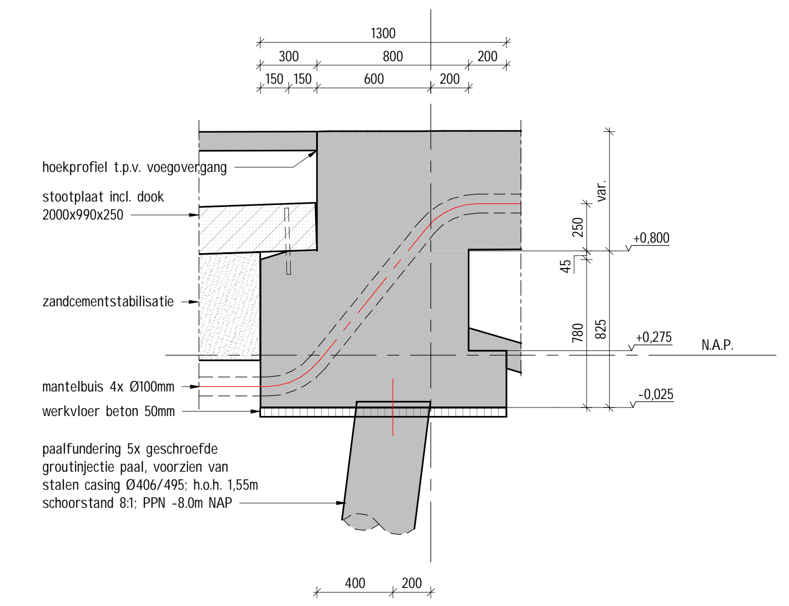
Detail 02 - landhoofd noord schaal 1 : 20
